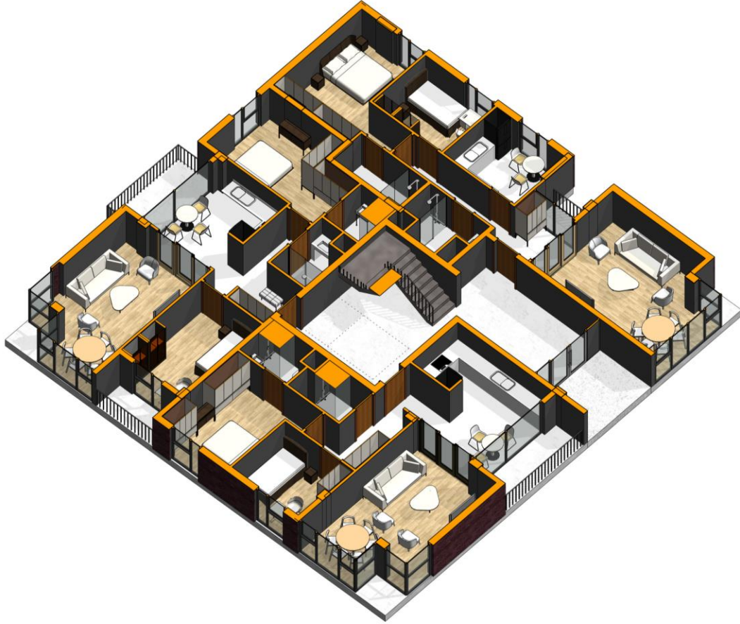
Kare Blok – Giriş Katı 3D Planı
