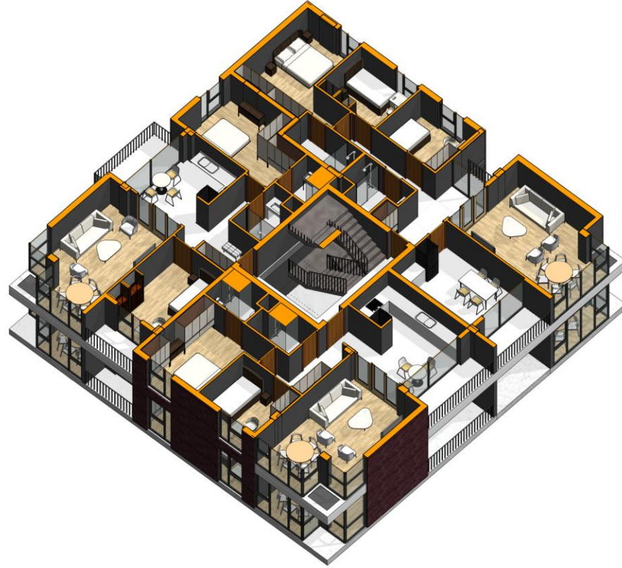
Kare Blok – Normal Kat 3D Planı
